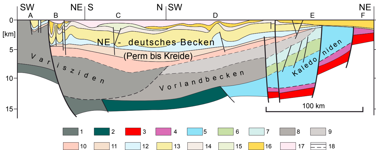
Abb. 3: Das Geopotential-Stockwerk I Mecklenburg-Vorpommerns ist tektonisch und sedimentär durch ein intrakontinentales Becken (NE-deutsches Becken) bestimmt (nach FRANKE, HOFFMANN & LINDERT 1996, S. 47, umgezeichnet u. vereinfacht, u. a. Profilverkürzung und Verzicht auf die Benennung der Störungen, s. dazu S. 46).
